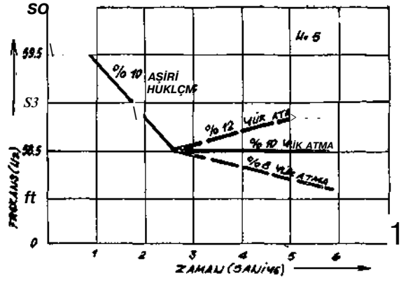
Değişik miktarlarda yük atma.
