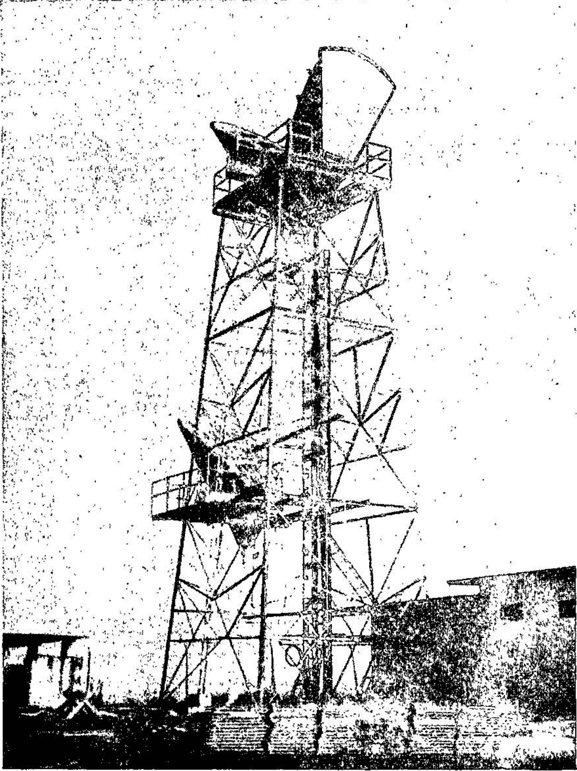
Malaya, Maxwell Hill'deki Microwave Radyo - link Anten ve Kulesi
