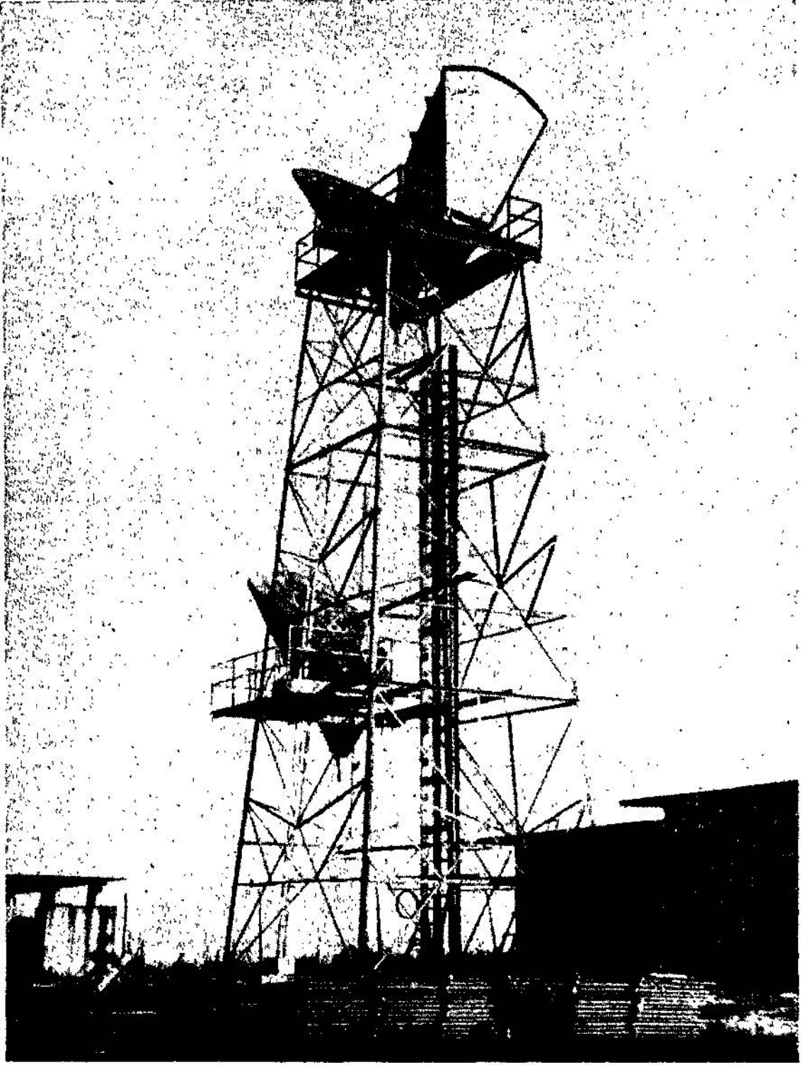
Malaya^ Maxwell Hill'deki Microvave Badyo - link Anten ve Kulesi
