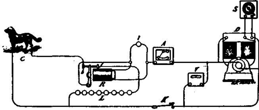
ŞEKİL 1. Harold P. Brown'un 1888'de deneylerinde AA ve DA'nın köpekler üzerindeki etkilerini incelemekte kullandığı devrelerden biri.
