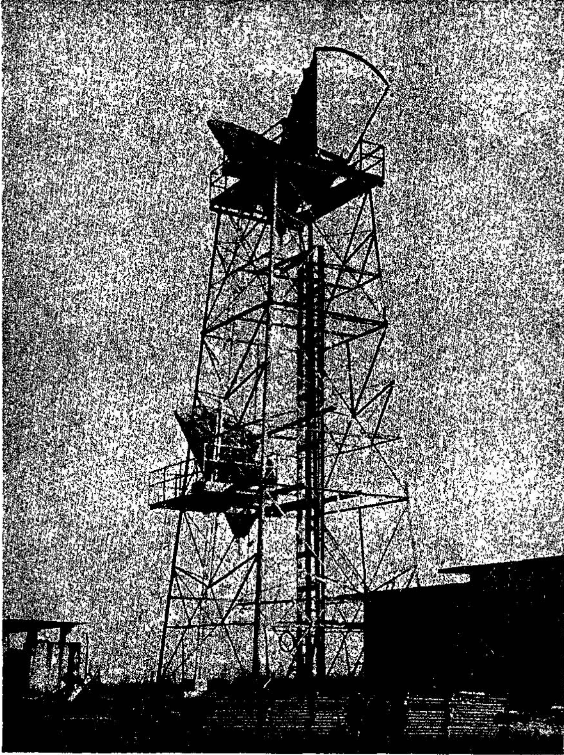
Malaya, Maxwell Hill'deki Microvave Radyo - link Anten ve Kulesi
