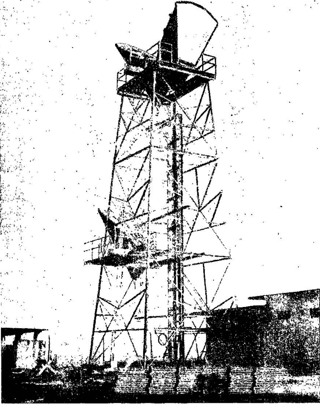
Malayà, Maxwell Hill'deki Microwave Radyo - link Anten ve Kulesi
