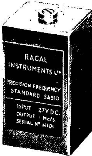
SA510 Hassas Frekans Standardı • StebUite 2 \times 10^{-6} • 1 Mc Çıkış
