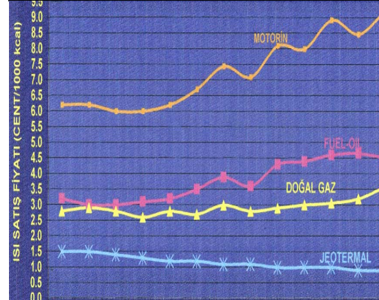
Şekil 1. JMIS ile diğer ısıtma sistemlerinin enerji maliyetlerinin karşılaştırılması
